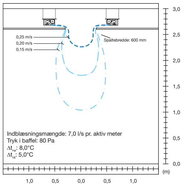
Figur 15 - 18. Lufthastigheder, frithængende ø-montage.
