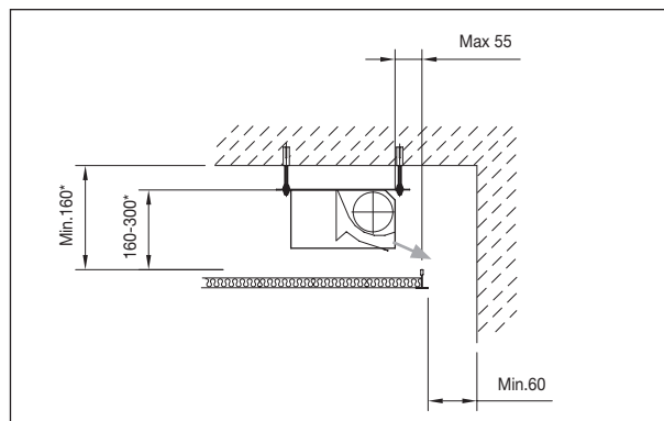
Figur 7. Mål ved installation, udløb langs væg.
