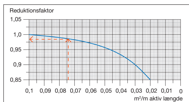
Diagram 5. Kapacitetsreduktion pga. minsket indløbsspalte.
