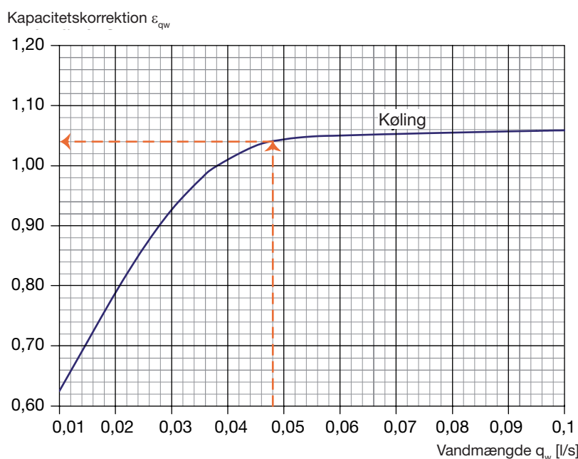
Diagram 3. Kapacitetskorrektion \varepsilon_{qw} for vandflow.
