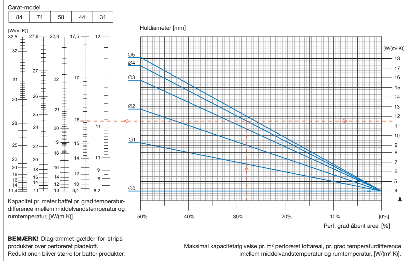
Diagram 1. Carat, kølekapaciteter ved montering over perforeret loft.
