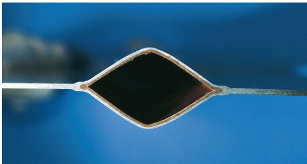
Billede 1. Tværsnit af Lindabs unikke strips. Den rombiske form giver en effektiv overflade.
